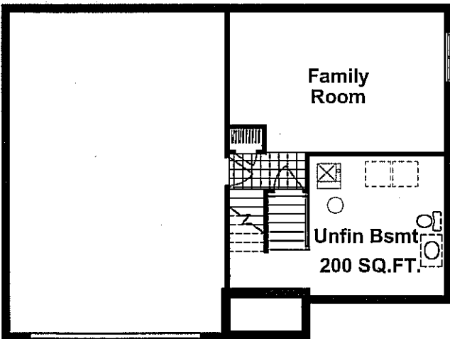
ELEV C
